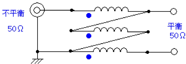
回路図
