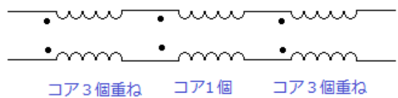
回路 キャンセル巻き
