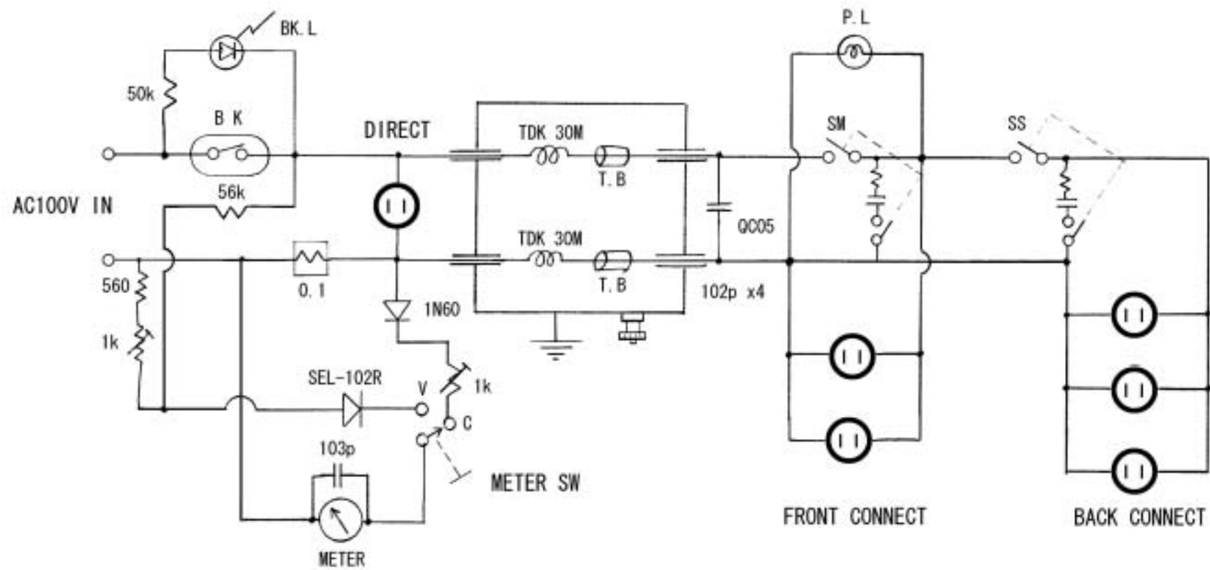
ADF-1 配線図
