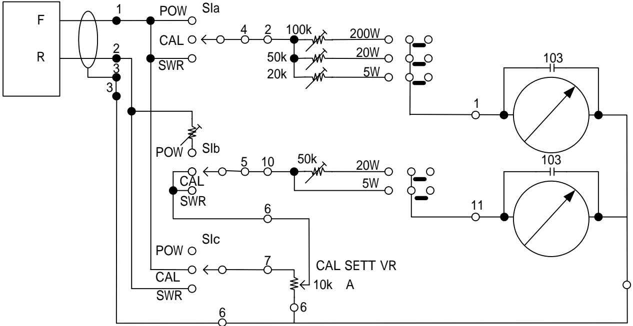
RW-32L回路图
