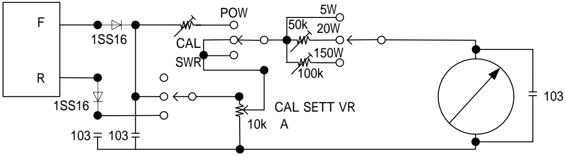
RW-31L回路图
